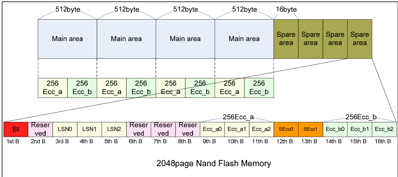
Figure 9-20 SECCSECTOR0~SECCSECTOR7
